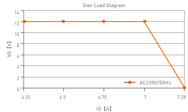
LM-75-12-G2D2
